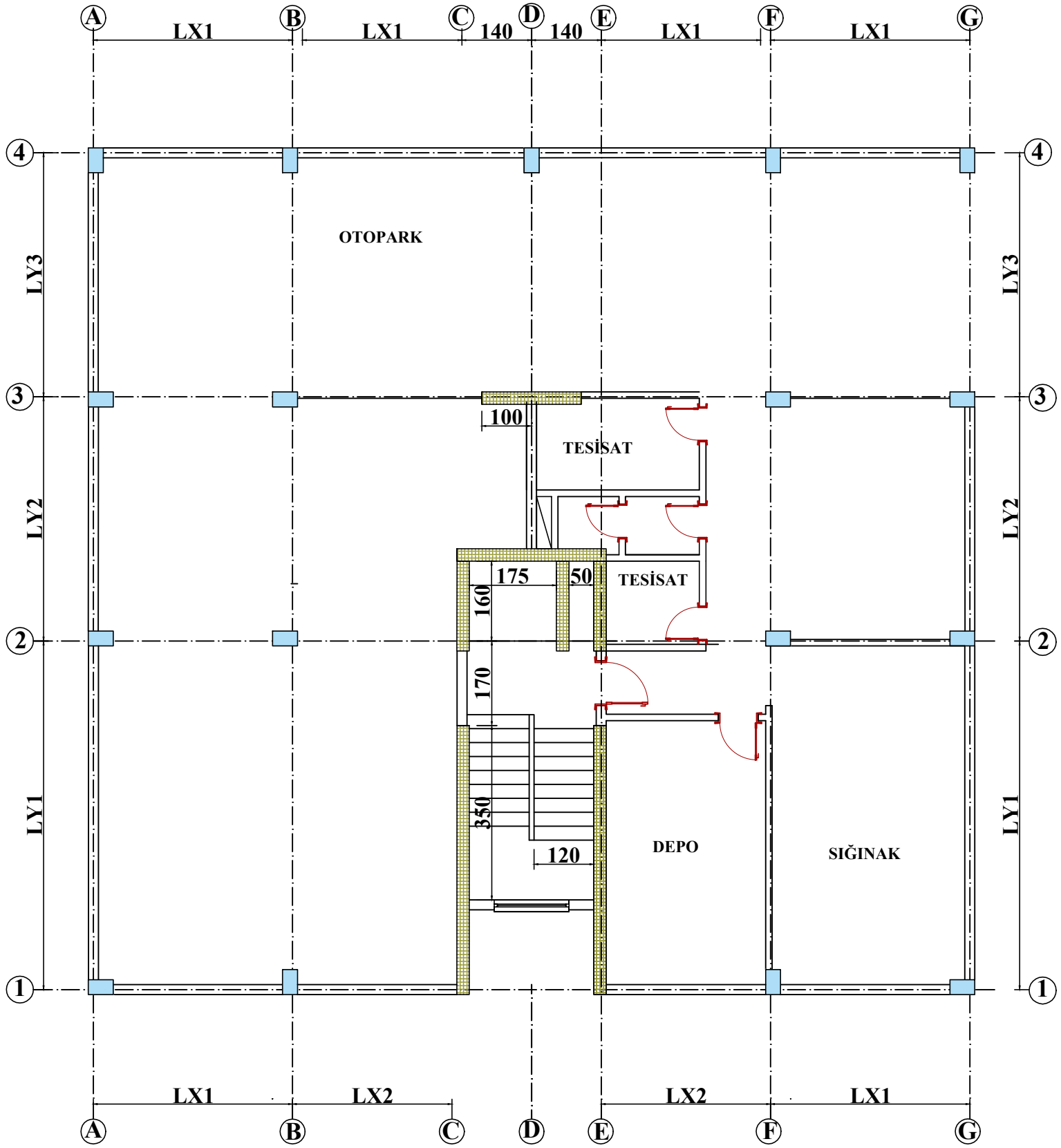
BODRUM KAT PLANI ÖLÇEK : 1/50
