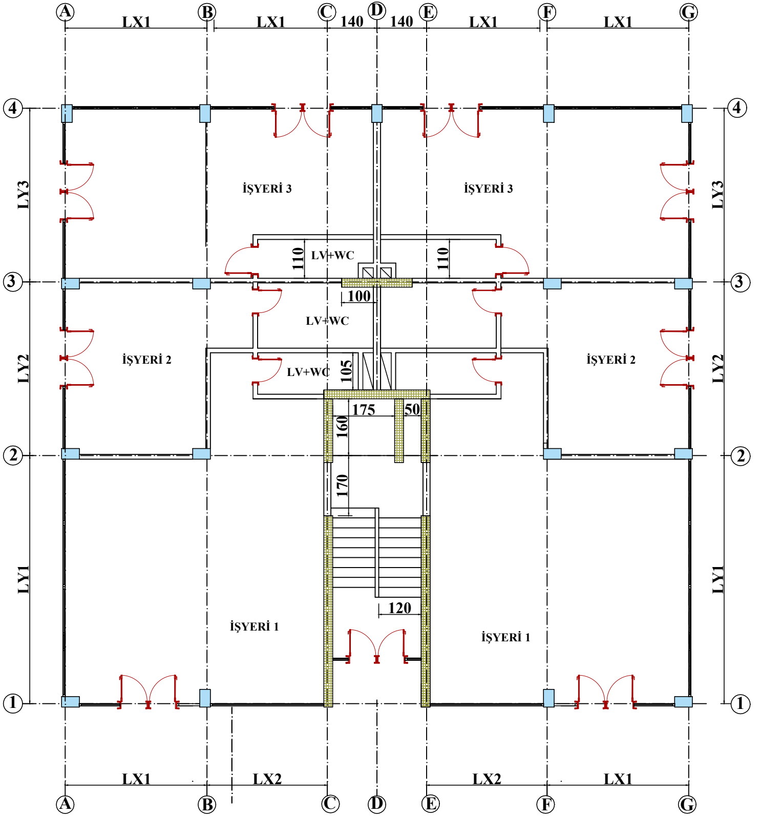
ZEMİN KAT PLANI ÖLÇEK : 1/50
