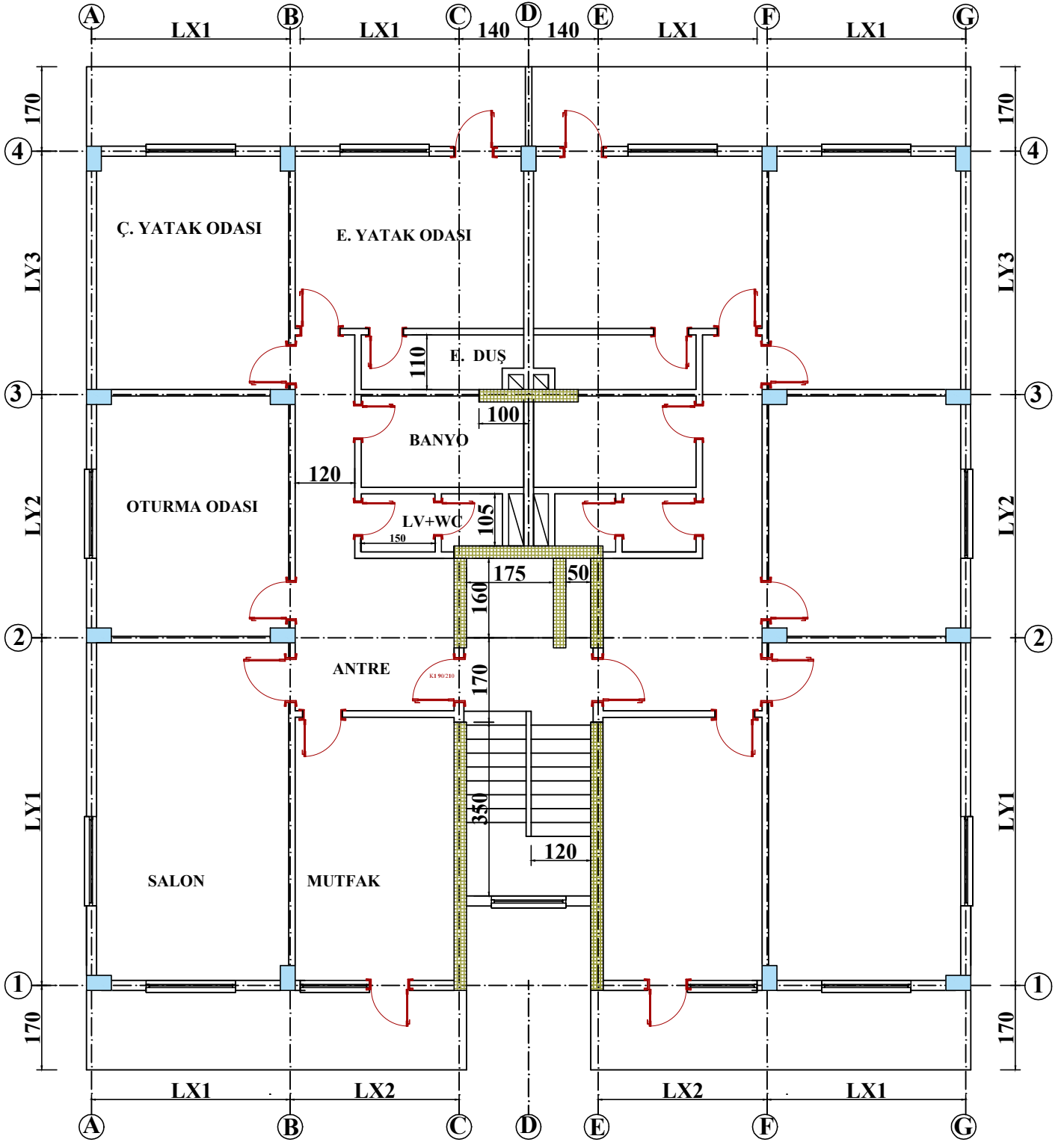
NORMAL KAT PLANI ÖLÇEK : 1/50
